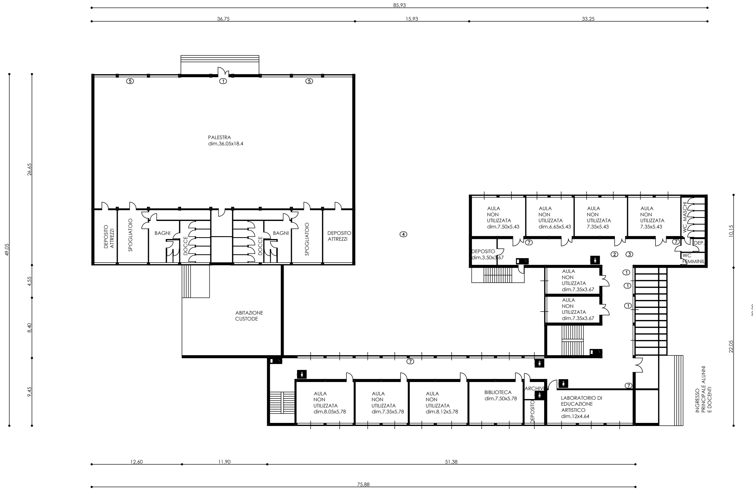
PIANTA PIANO TERRA Scala 1:250
